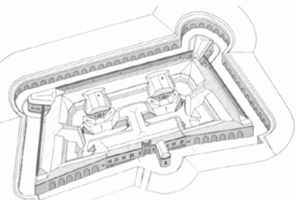
Pruski fort pośredni z lat 70. XIX wieku
