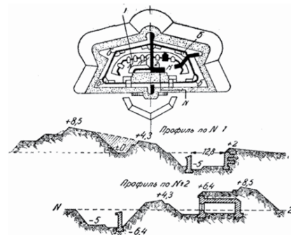
Plan rosyjskiego standardowego fortu głównego z 1879 r. (F-1879)
